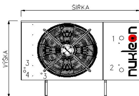
ČELNÍ POHLED
